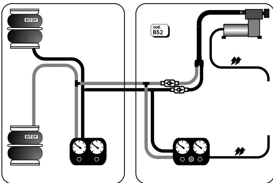
SCHEMA DI MONTAGGIO DEL B52
